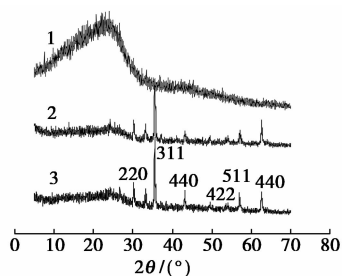
1—SJC; 2— 300^\circ\text{C} 下 \text{Fe}_3\text{O}_4 @SJC; 3— 500^\circ\text{C} 下 \text{Fe}_3\text{O}_4 @SJC
