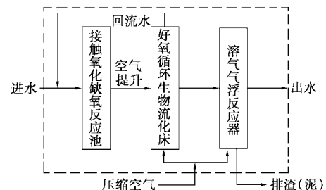
图 3 HSBCR 工艺流程示意图
