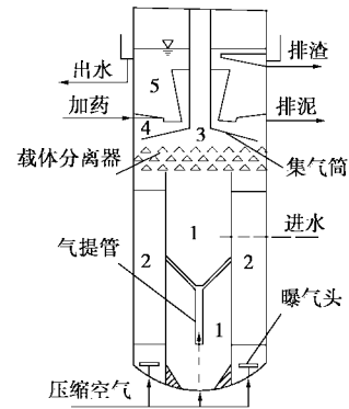
1—缺氧反应区;2—好氧流化反应区;3—气体收集区; 4—泥水上升区;5—气浮澄清区
