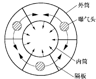
图 2 反应区平面示意图
