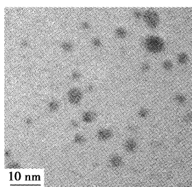
图2 SH10还原 [\text{Ag}(\text{NH}_3)_2]^+ 得到银纳米粒子的HRTEM
