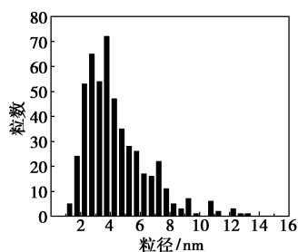
图3 银纳米粒子的粒径分布
