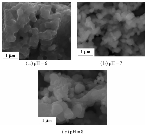
图 2 不同 \text{pH} 条件下合成的 \text{Li}_{1.2}\text{Ni}_{0.2}\text{Mn}_{0.6}\text{O}_2 扫描电镜图片
