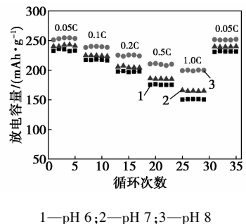
图 4 不同 \text{pH} 条件下合成的 \text{Li}_{1.2}\text{Ni}_{0.2}\text{Mn}_{0.6}\text{O}_2 倍率放电容量
