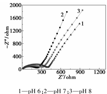
图 5 不同 \text{pH} 条件下合成的 \text{Li}_{1.2}\text{Ni}_{0.2}\text{Mn}_{0.6}\text{O}_2 半电池的交流阻抗
