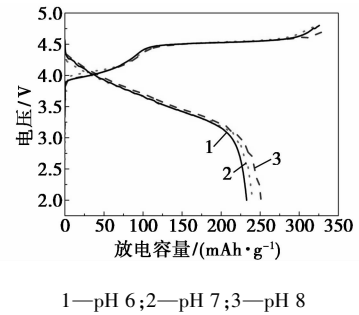
图 3 不同 \text{pH} 条件下合成的 \text{Li}_{1.2}\text{Ni}_{0.2}\text{Mn}_{0.6}\text{O}_2 首次充放电曲线
