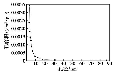
图3 中空碳纳米纤维的介孔孔径分布
