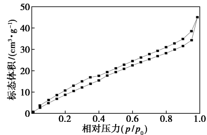
图2 中空碳纳米纤维的氮气吸附与脱附等温线
